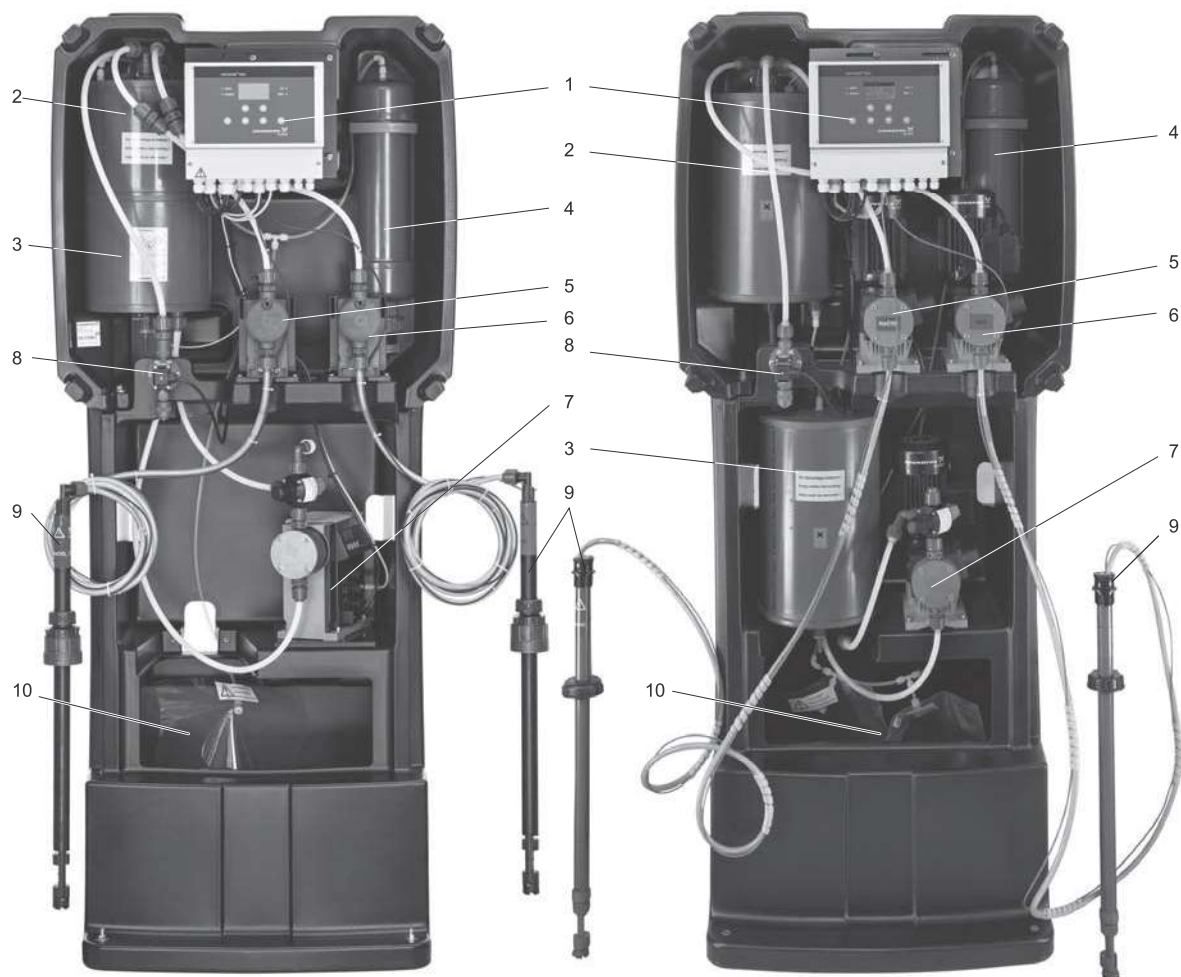
7. ábra OCD-162-30 (bal) és OCD-162-60 (jobb) fedél nélkül
